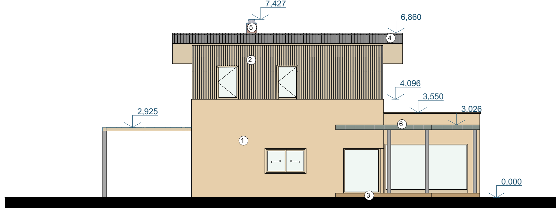
SEVERNÍ POHLED (1:100)
