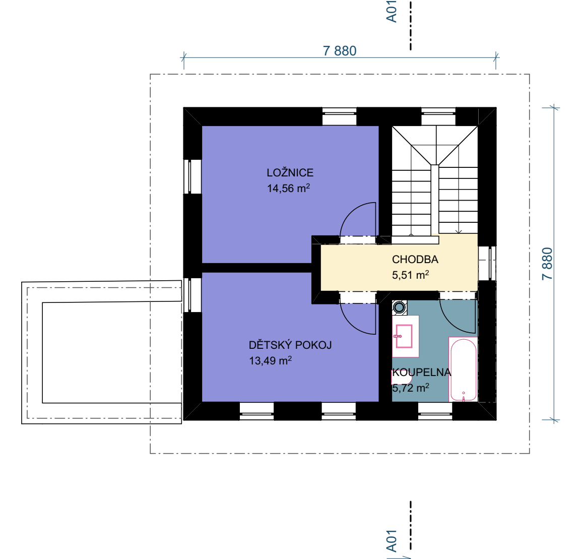
PŮDORYS 2.NP (1:100)
