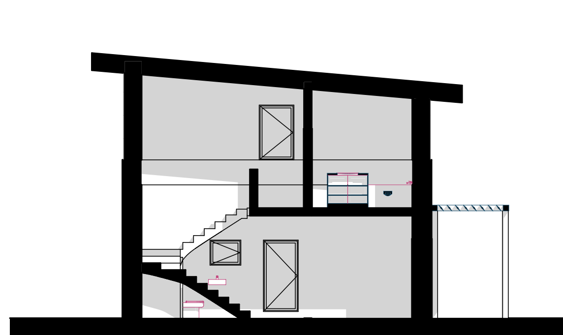
ŘEZ A01 (1:100)
